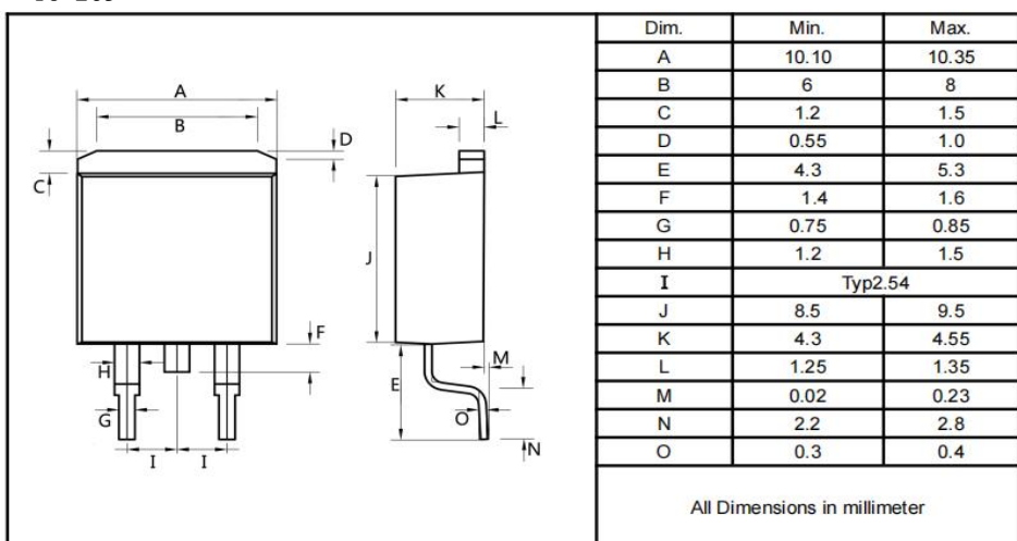
TO-263
